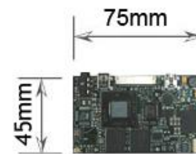
Mobile-ITX
